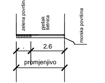
KARAKTERISTIČAN POPREČNI PRESJEK B - B, MJ. 1:200
