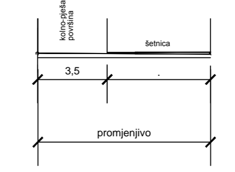
KARAKTERISTIČAN POPREČNI PRESJEK A - A, MJ. 1:200
